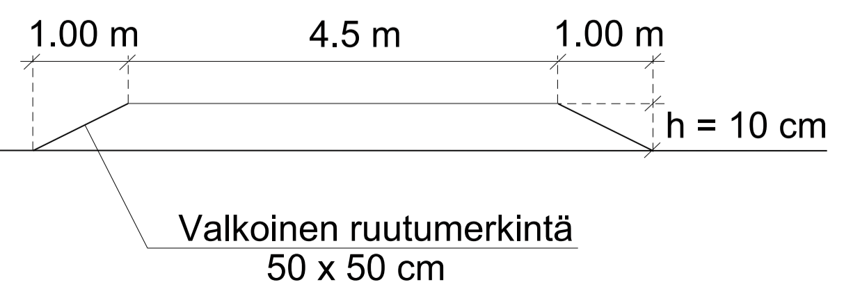
LEIKKAUS A - A, KOROTETTU SUOJATIE
