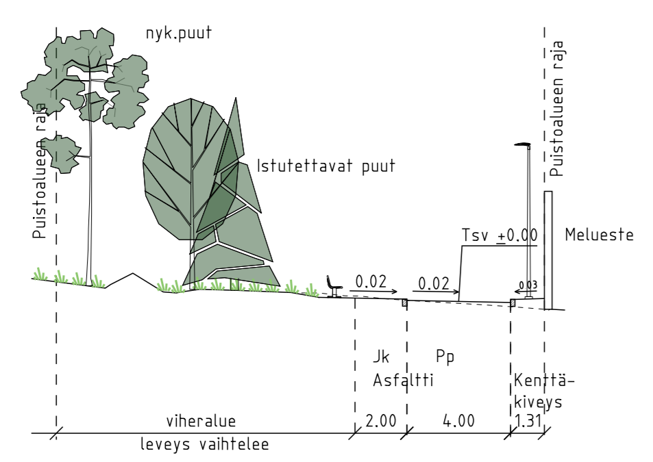
POIKKILEIKKAUS A-A PL. 75 1:200
