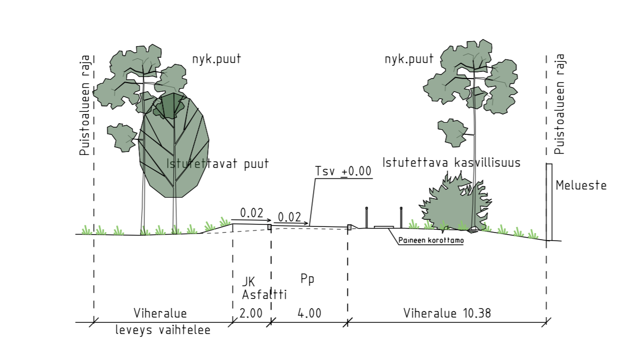
POIKKILEIKKAUS B-B PL. 140 1:200
