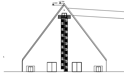
JULKISIVÄ LUODE
