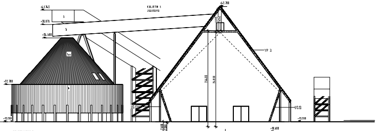
PÄÄNULIIVITUKKOS JULKISIVU
