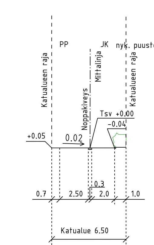
ADJUTANTINPOLKU POIKKILEIKKAUS G-G 1:200
