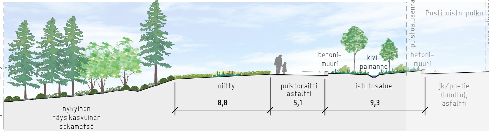
Postipuisto Leikkaus A - A, 1:200
