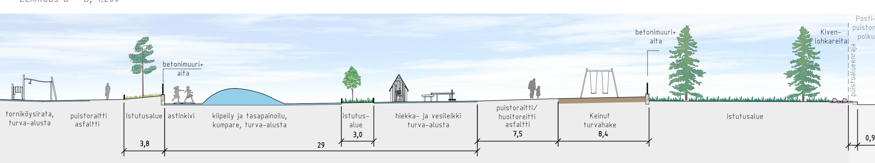
Postipuisto Leikkaus B - B, 1:200
