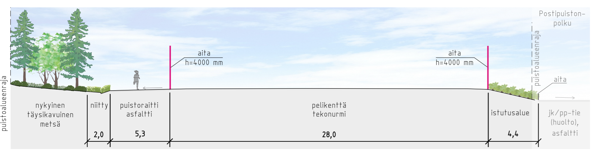
Postipuisto Leikkaus C - C, 1:200
