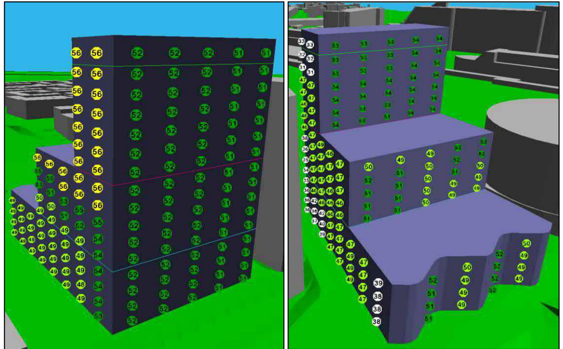
Kuva 14. Laivamelusta aiheutuvat yöajan keskiäänitasot L_{A,eq22-7} toimisto-, liiketila- ja hotellikerrosten julkisivulla
