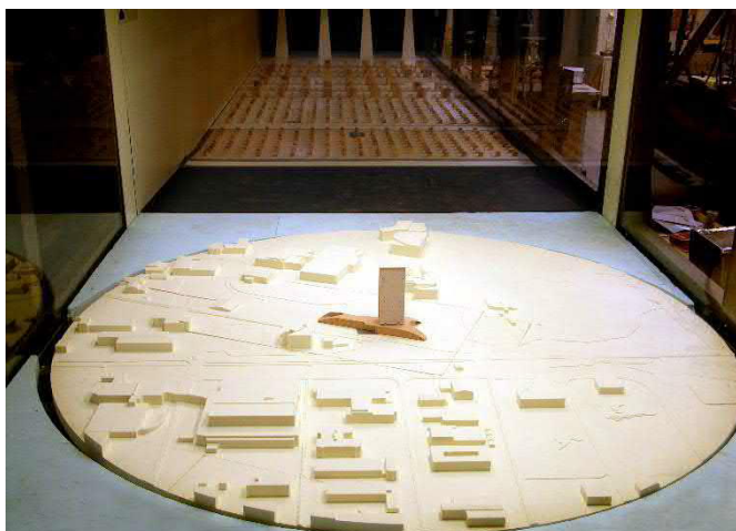
Kuva L3.2: Esimerkki Konsultin rajakerros-tuulitunnelikoekeesta vuodelta 2008 ("Føniks", Stavanger, Norja). Rakennuksen havainnekuvan reiät osoittavat pisteitä, joihin pinta-asennetut paineanturit on sijoitettu.
