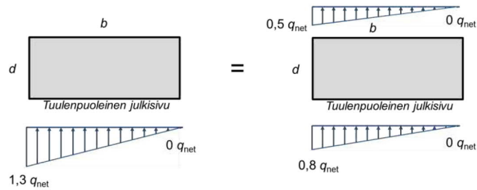
Kuva L4.1 Kuormitustapaukset tuulikuorman vääntövaikutusten tarkasteluun. Kuvassa q_{net} = tämän raportin mukaisesti määritetty kokonaistuulikuorma.
