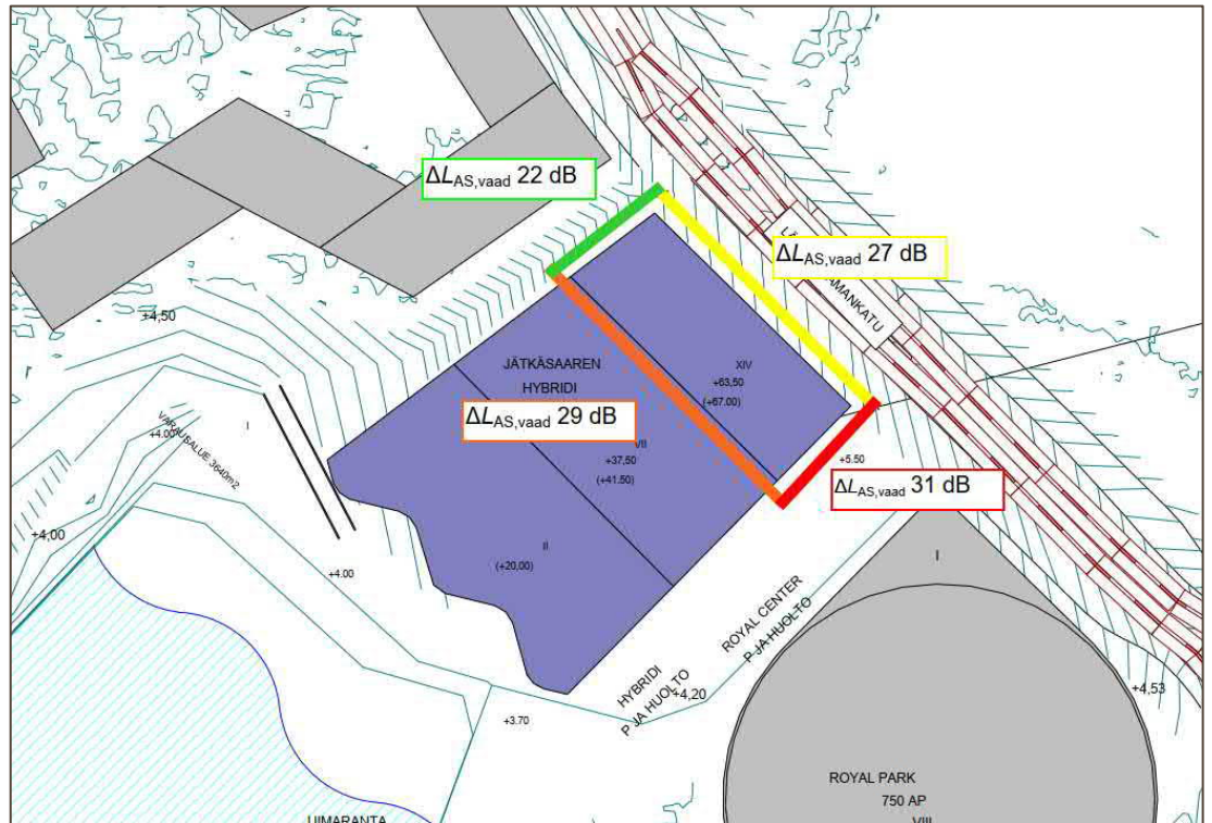
Kuva 23. Hotellikerrosten äänitasoerosuositukset \Delta L_{A,vaad} laivamelua vastaan julkisivuittain (laivamelu mitoittava).
