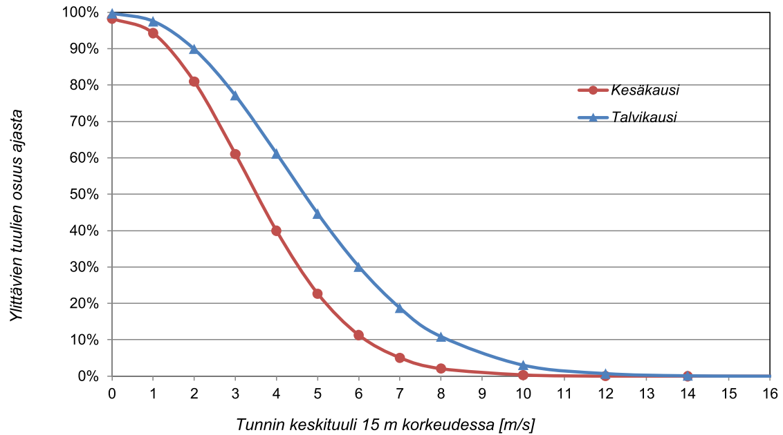
Tuulisuuden perustaso kohdealueessa (15 m korkeus)
