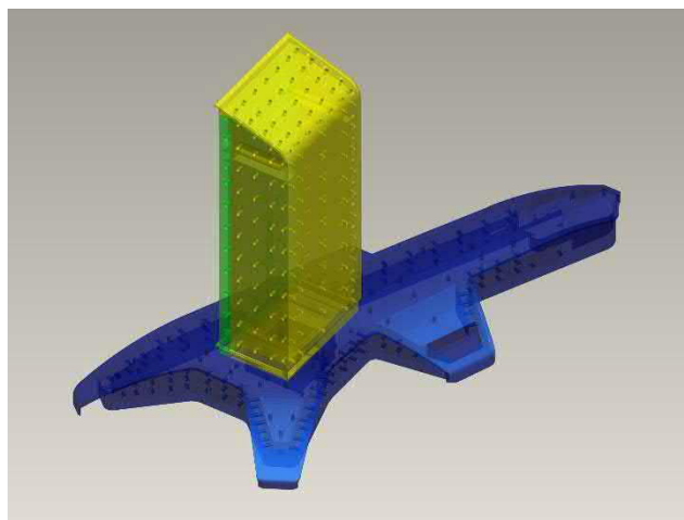
Kuva L3.2: Esimerkki Konsultin rajakerros-tuulitunnelikoekeesta vuodelta 2008 ("Føniks", Stavanger, Norja). Rakennuksen havainnekuvan reiät osoittavat pisteitä, joihin pinta-asennetut paineanturit on sijoitettu.
