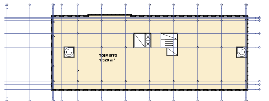
Kerros 05
