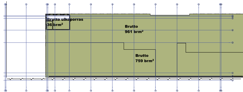
Kellari K1
