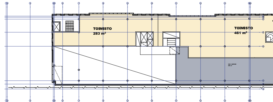
Kerros 01
