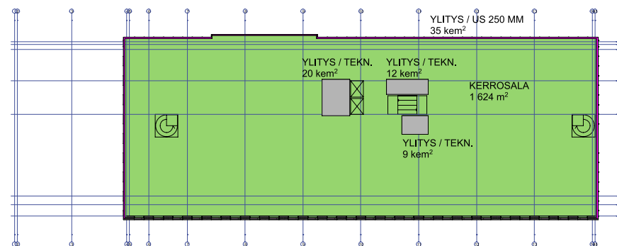
Kerros 06
