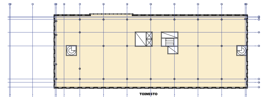
Kerros 06
