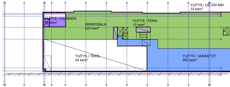
Kerros 01
