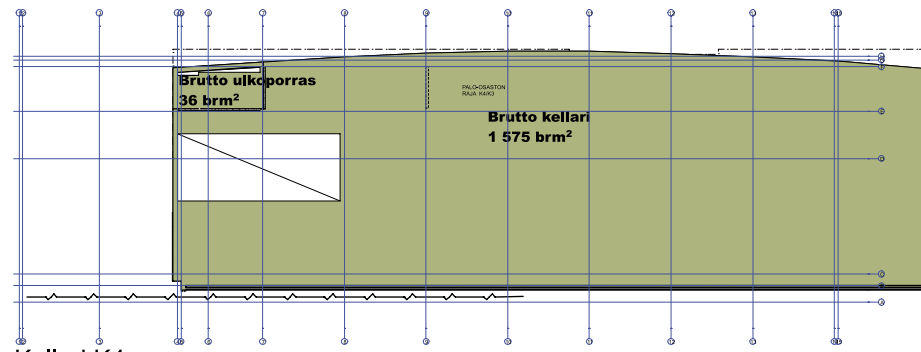
Kellari K4
