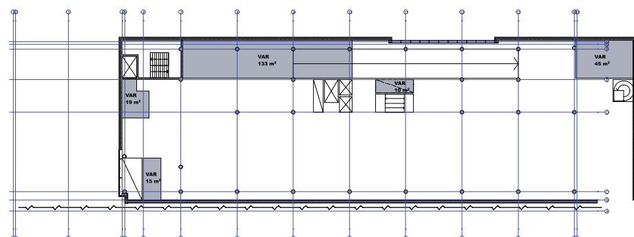
Kellari K2
