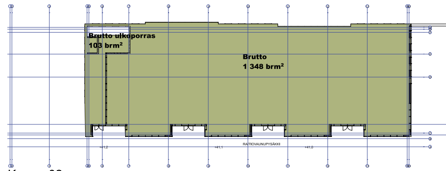
Kerros 02
