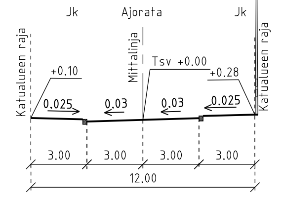
POIKKILEIKKAUS K-K 1:200
