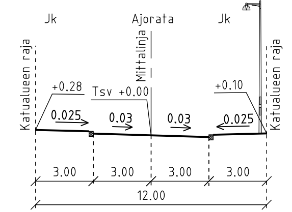
POIKKILEIKKAUS H-H 1:200
