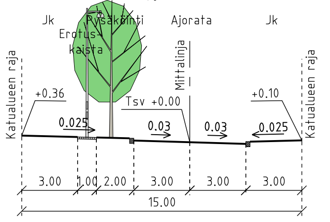
POIKKILEIKKAUS J-J 1:200
