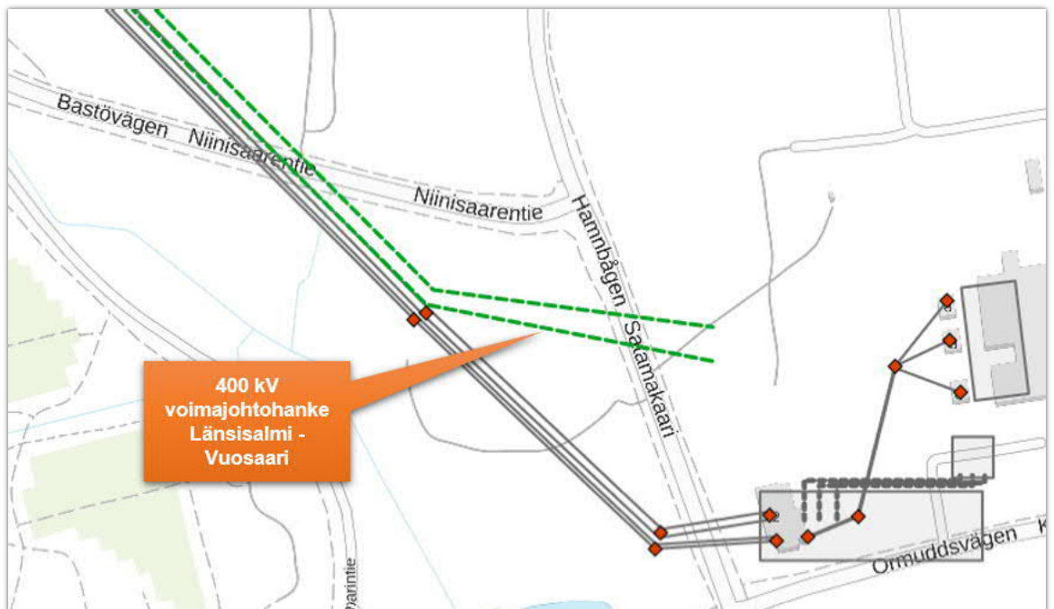
Kuva 1. Voimajohdot asemakaava-alueella.
