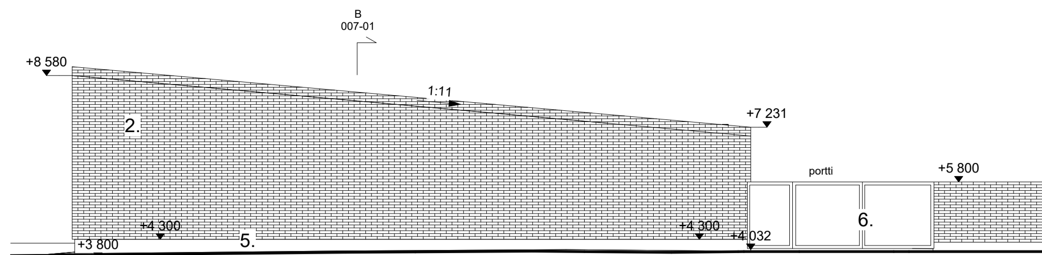
Julkisivu itään 1 : 100
