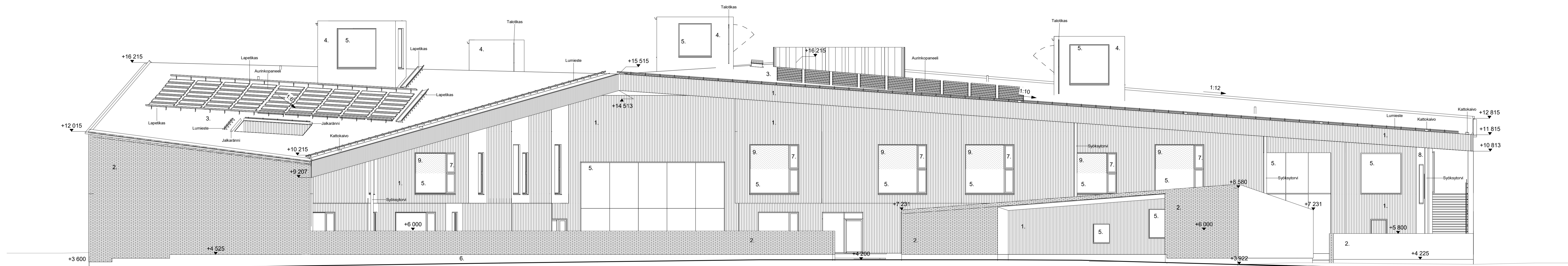
Julkisivu etelään 1 : 100
