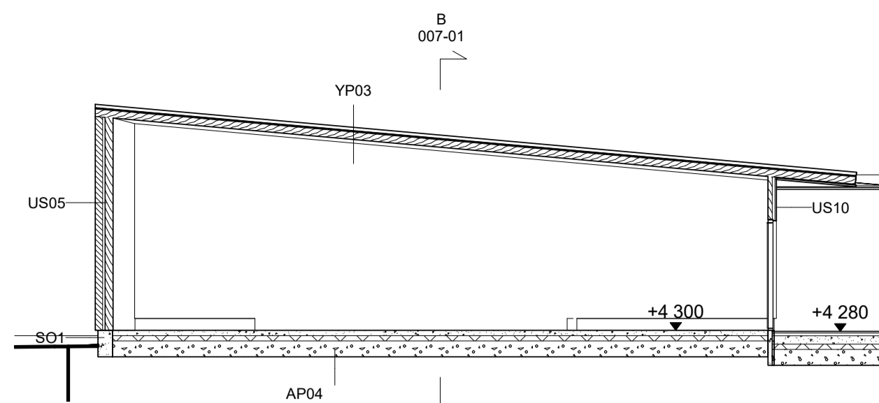
Leikkaus a-a, piharakennus 1 : 100
