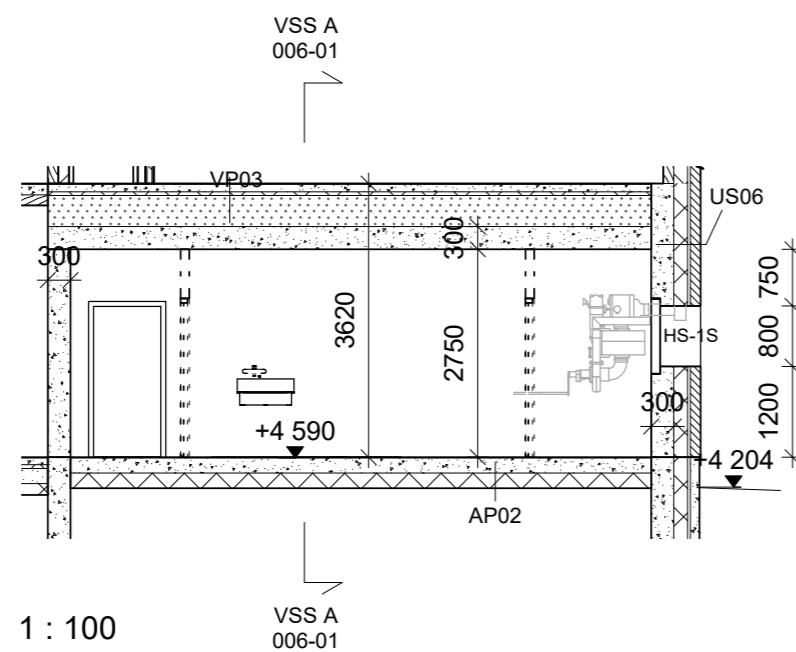
A-A 1 : 100
