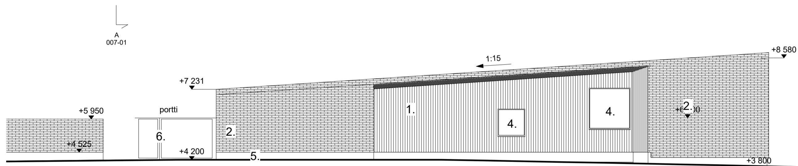
Julkisivu etelään 1 : 100
