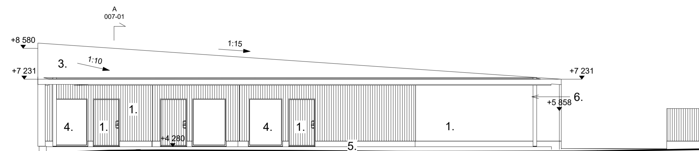
Julkisivu pohjoiseen 1 : 100
