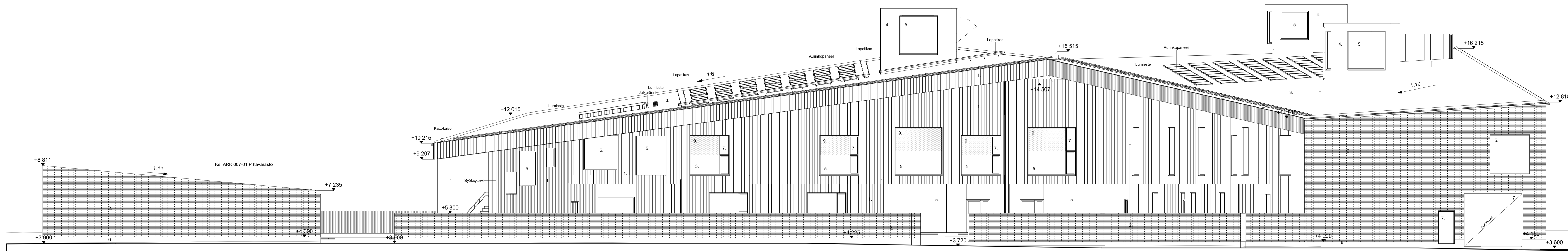
Julkisivu itään 1 : 100
