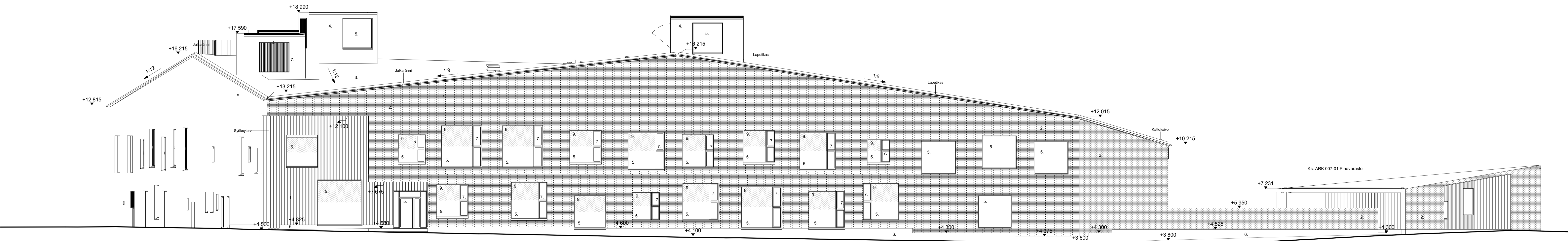
Julkisivu länteen 1 : 100
