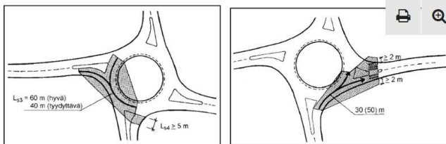
Tiehallinto, Tasoliittymät, S. 47 Kuva 5.7 Näkemien mitoitus edellisen tulohaaran suuntaan. Kuva 5.8 Näkemät ajosuuntaan.
