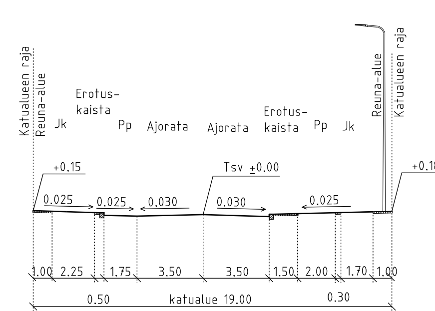
METSÄPURONTIE, ITÄ E-E
