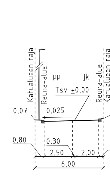
RAITTI VÄLILLÄ LAMPUOTILANTIE-PAKILANTIE I-I
