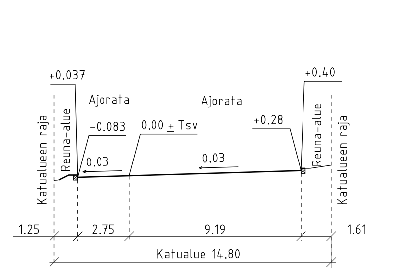
LAMPUOTILANTIE KÄÄNTÖPAIKKA F-F
