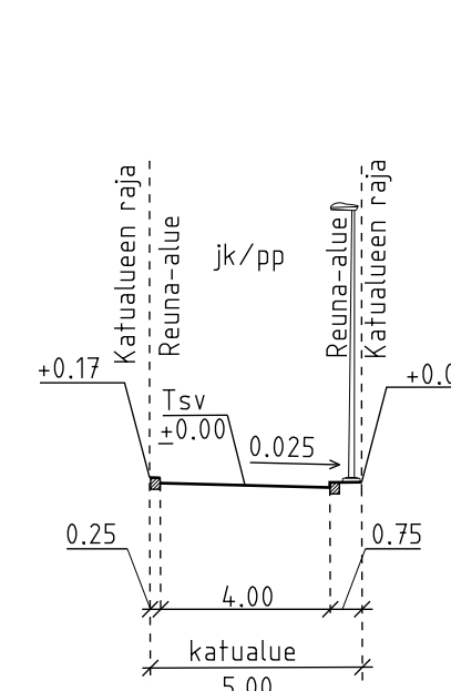
LAMPUOTILANTIE RAITTI Välillä Lamputilantie - Maunulantie G-G
