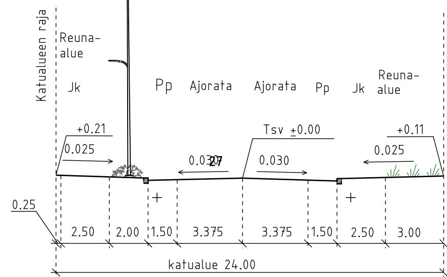
METSÄPURONTIE, LÄNSI D-D
