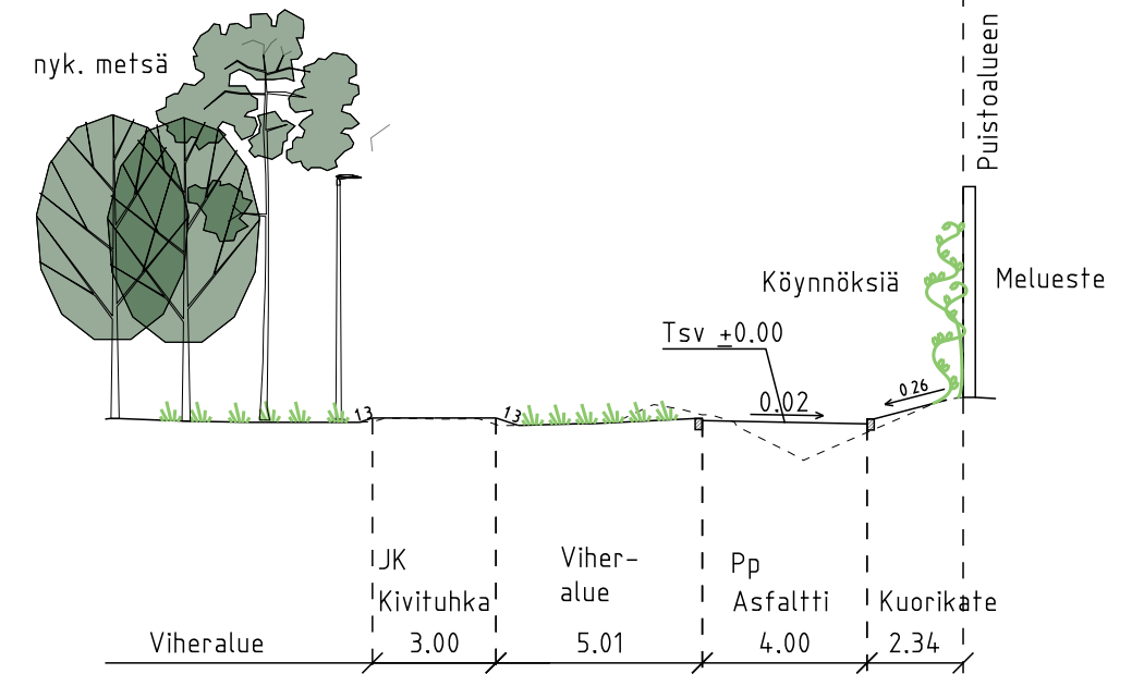
POIKKILEIKKAUS E-E PL. 735 1:200
