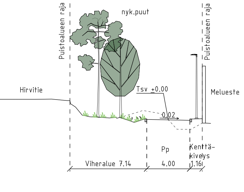
POIKKILEIKKAUS D-D PL. 530 1:200
