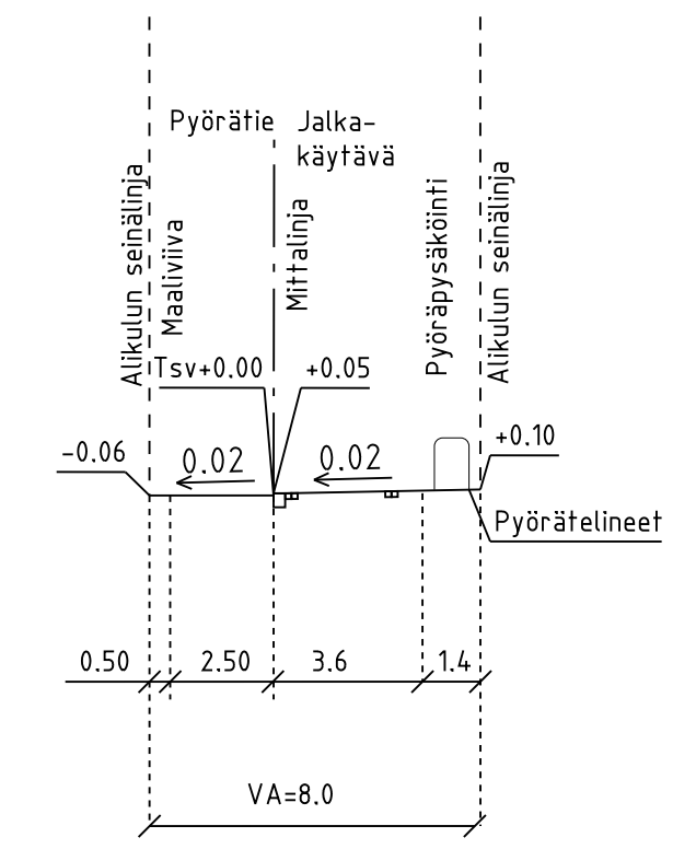
UKKO-PEKAN PORTAAN ALIKULKU POIKKILEIKKAUS E-E 1:200
