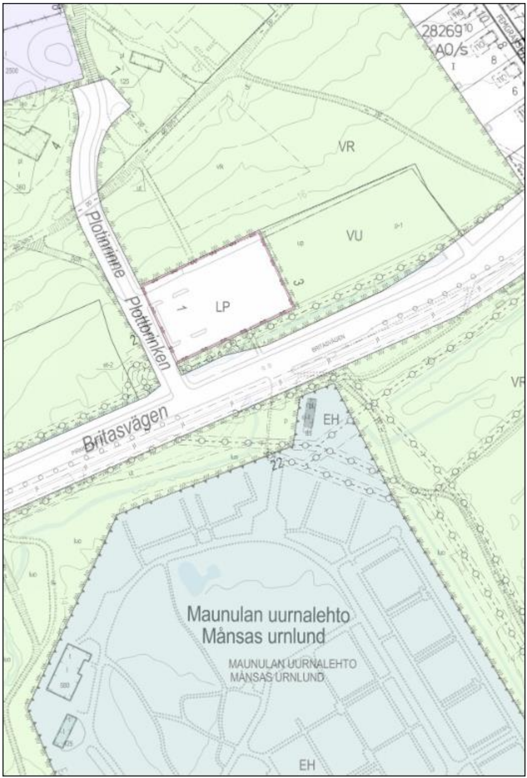
Raide-Jokerin Pirkkolantien sähkönsyöttöasema, ote ajantasa-asemakaavasta.
