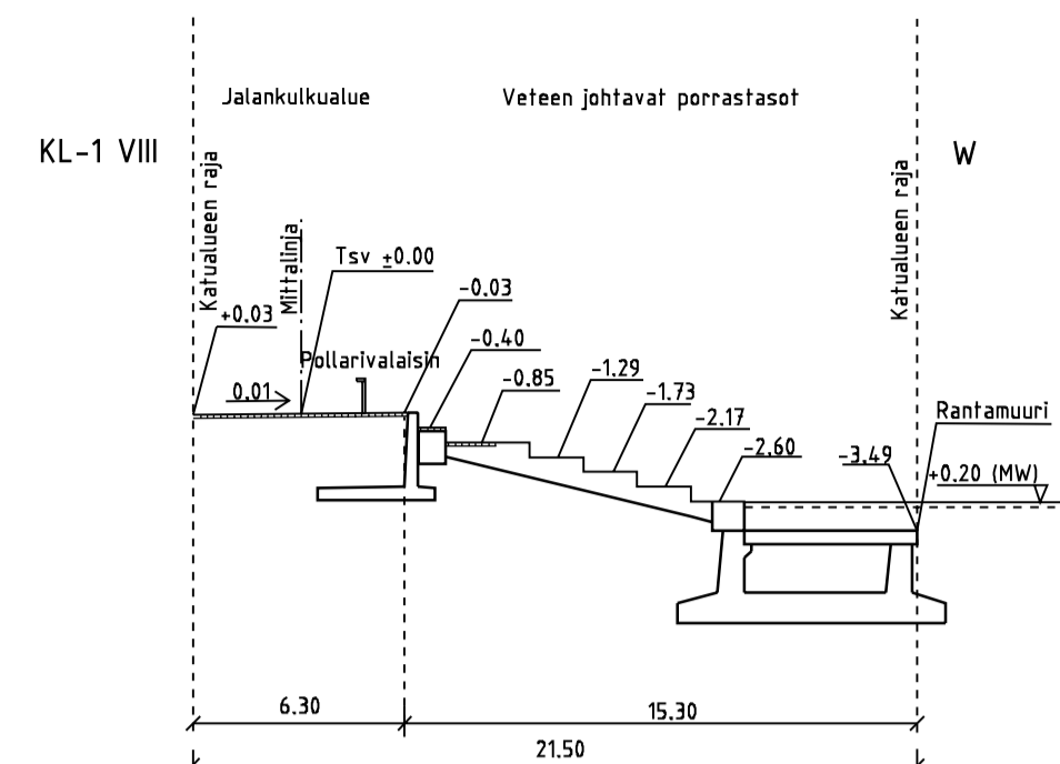
POIKKILEIKKAUS C-C 1:200
