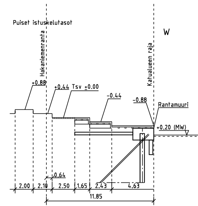
POIKKILEIKKAUS A-A 1:200
