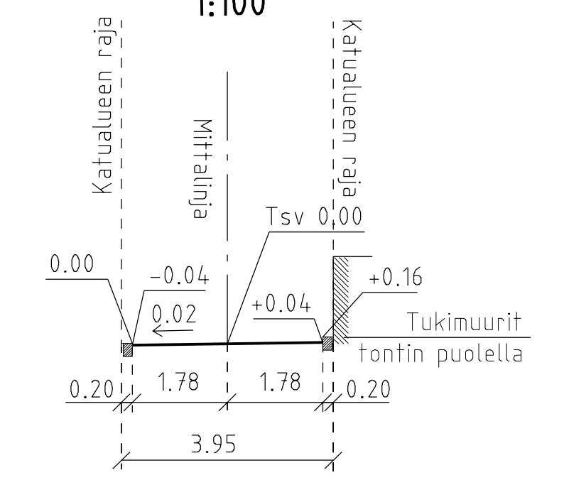
POIKKILEIKKAUS C-C 1:100
