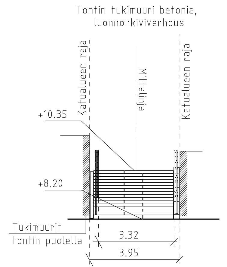
POIKKILEIKKAUS B-B 1:100
