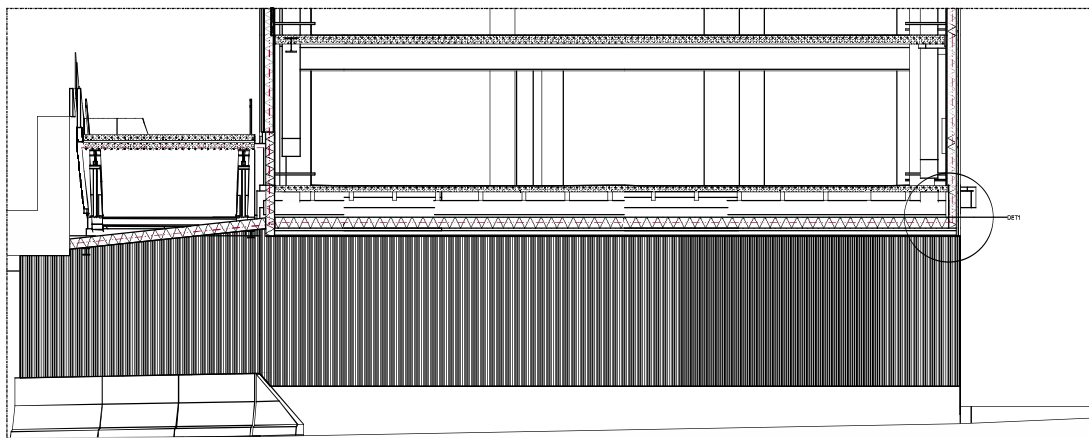
LEIKKAUS A-A, KAISTOJEN VÄLINEN OSASTONVA SEINÄ
