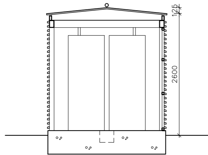
LEIKKAUS A-A
