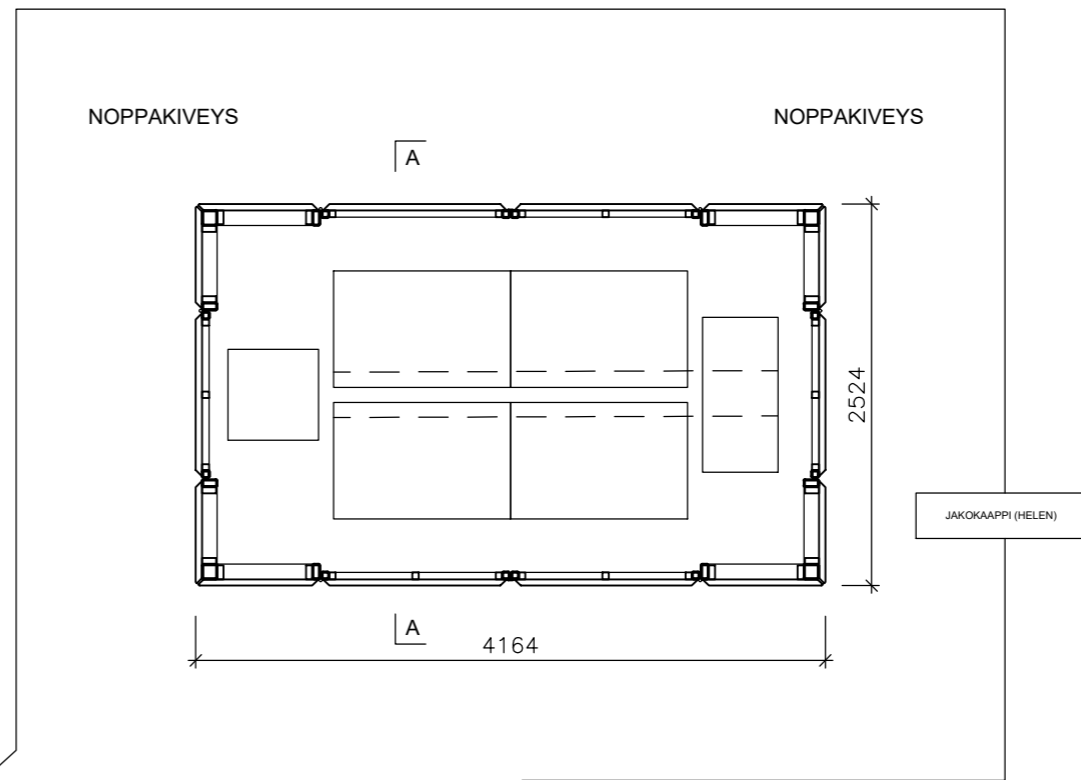
POHJAPIIRUSTUS
