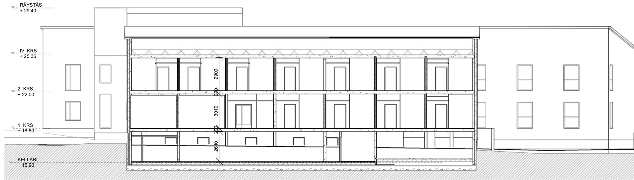
LEIKKAUS B-B 1 : 200
