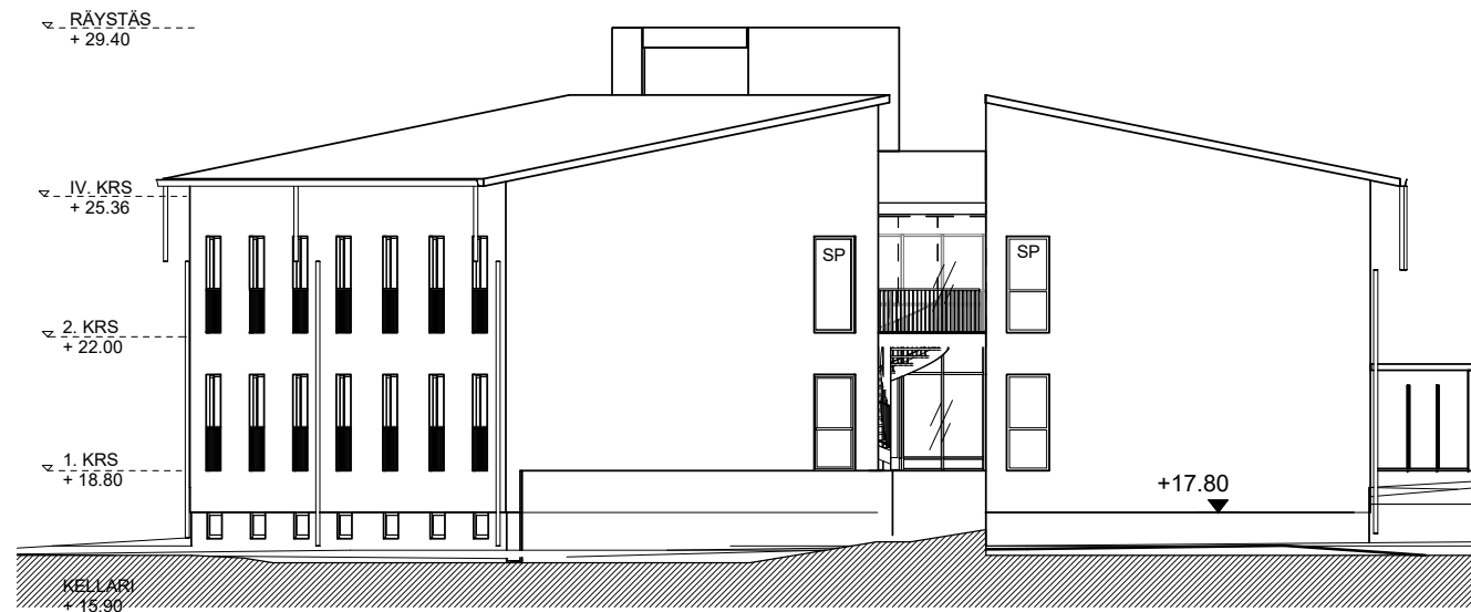
Julkisivu ETELÄÄN 1 : 200
