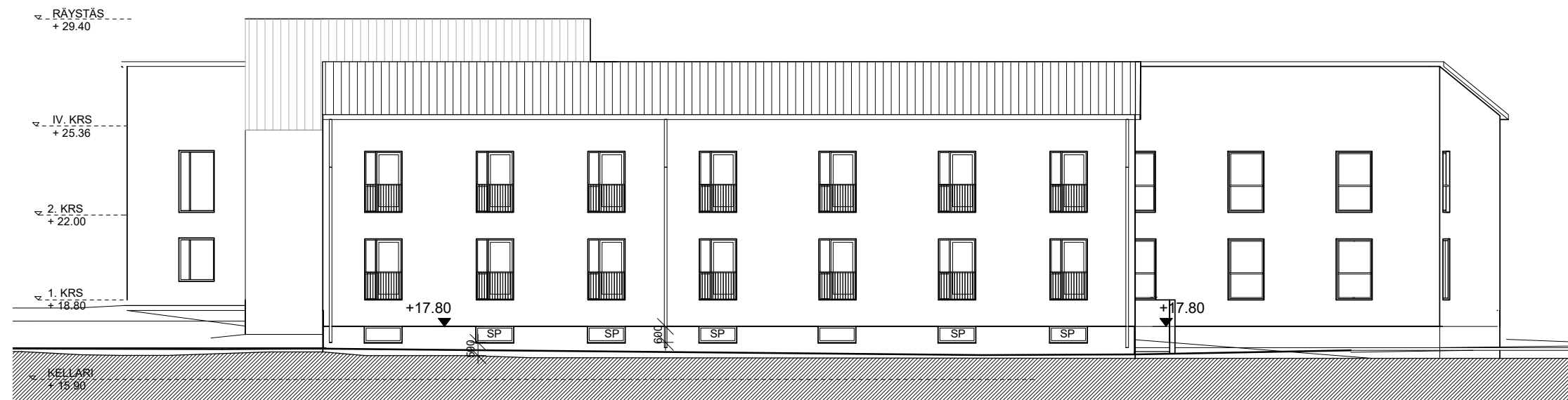
Julkisivu LÄNTEEN 1 : 200
