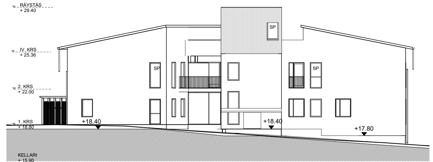
Julkisivu POHJOISEEN 1 : 200
