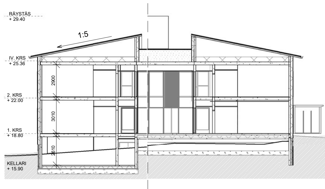
LEIKKAUS A-A 1 : 200
