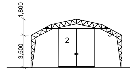
LEIKKAUS A-A
