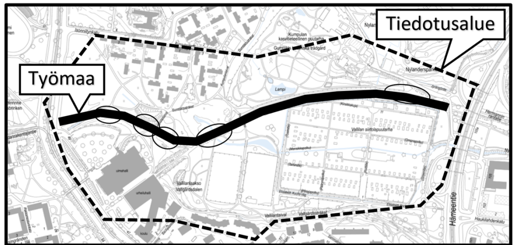
Kuva 1. Työmaan sijainti ja tiedotusalue (Määräys 4). Louhinta-, paalutus-, pontitus- ja ankkurointikohteet on ympyröity.
