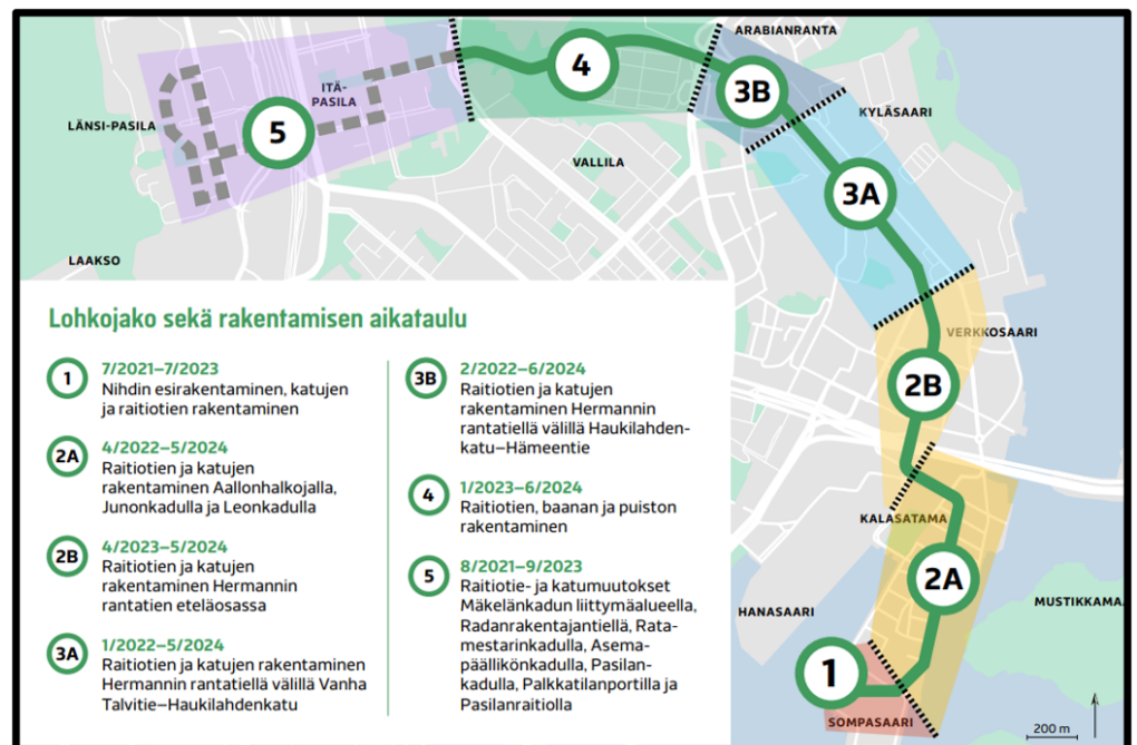
Kuva 2. Kalasadamasta Pasilaan -hankkeen lohkot ja niiden rakennusaikataulut.
