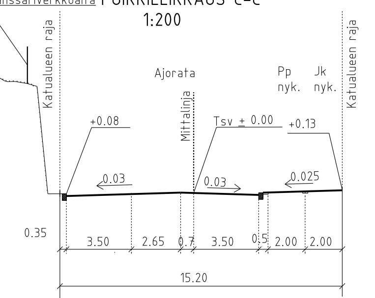
Panssariverkkoaita POIKKILEIKKAUS C-C 1:200
