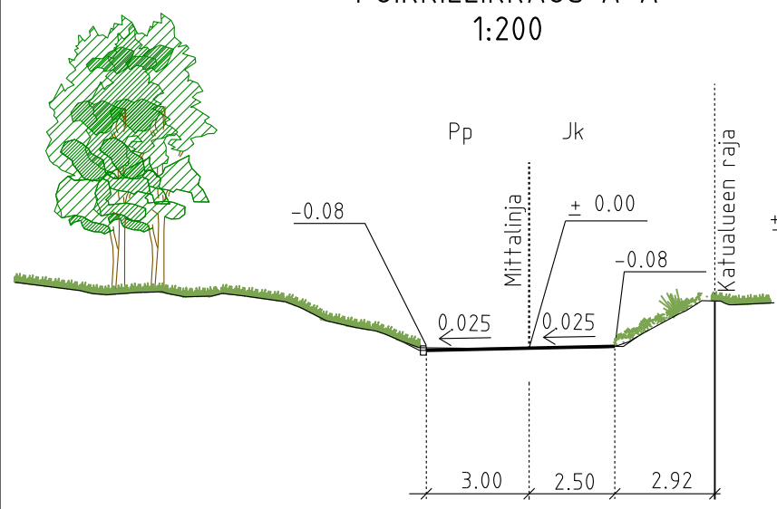
POIKKILEIKKAUS A-A 1:200
