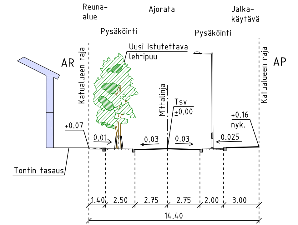
HARBONKATU POIKKILEIKKAUS A-A 1:200
