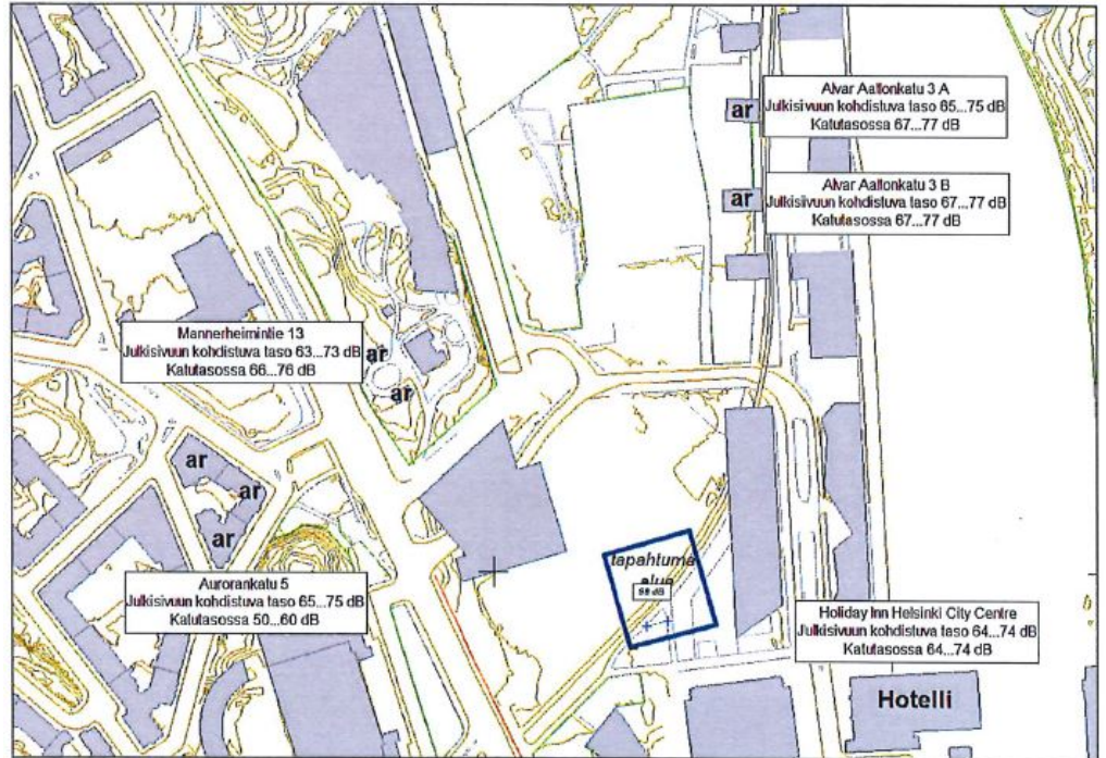
Kuva 4. Melutasot lähimpien altistuvien kohteiden julkisivuilla ja katutasossa julkisivujen edessä, kun äänentaso on miksausasteessa (FOH) säädetty LpA = 98 dB
