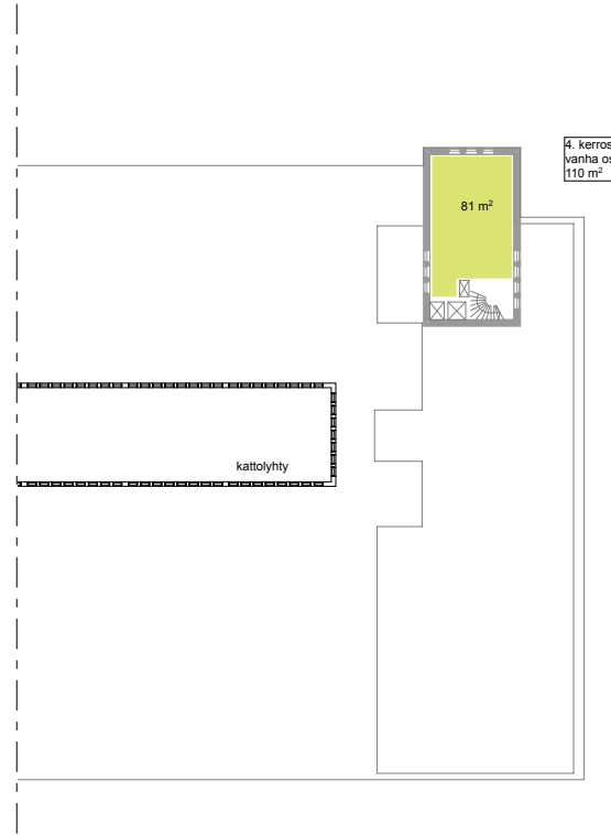
4.kerros 1 : 750
