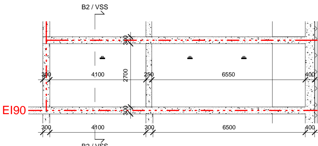
LEIKKAUS A1/VSS
