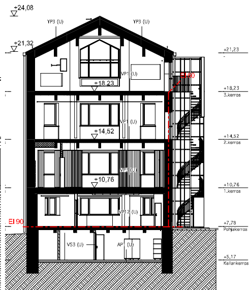
004.003 Leikkaus D 1:100
