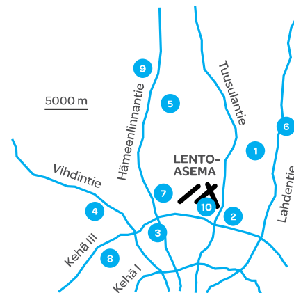
Kuva 38. Kiinteät melumittausasemat Helsinki-Vantaan ympäristössä.
