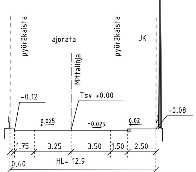
HOPEASALMENTIEN SILTA POIKKILEIKKAUS H-H 1:200
