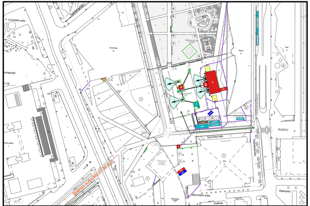
Kuva 1. Esiintymislavan sijainti ja kaiuttimien suuntaus.
