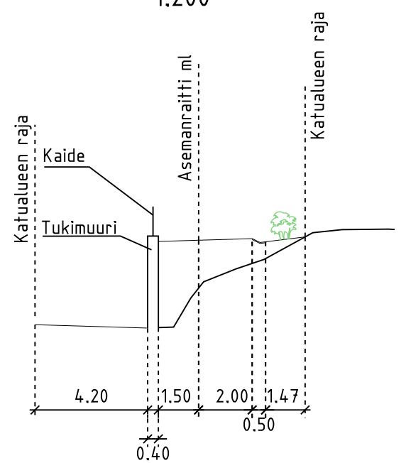
POIKKILEIKKAUS A - A 1:200
