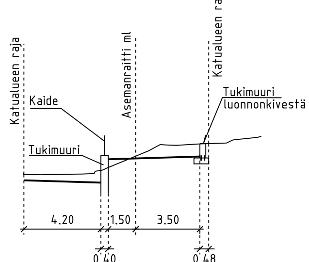
POIKKILEIKKAUS B - B 1:200
