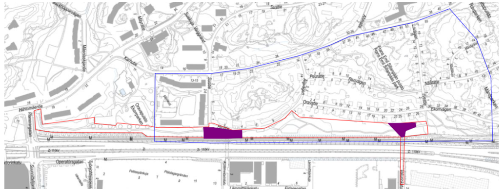
Kuva 1. Tiedotusalue rajattu sinisellä viivalla, työmaa-alue punaisella viivalla ja violetin värillä meluavat työkohteet.
