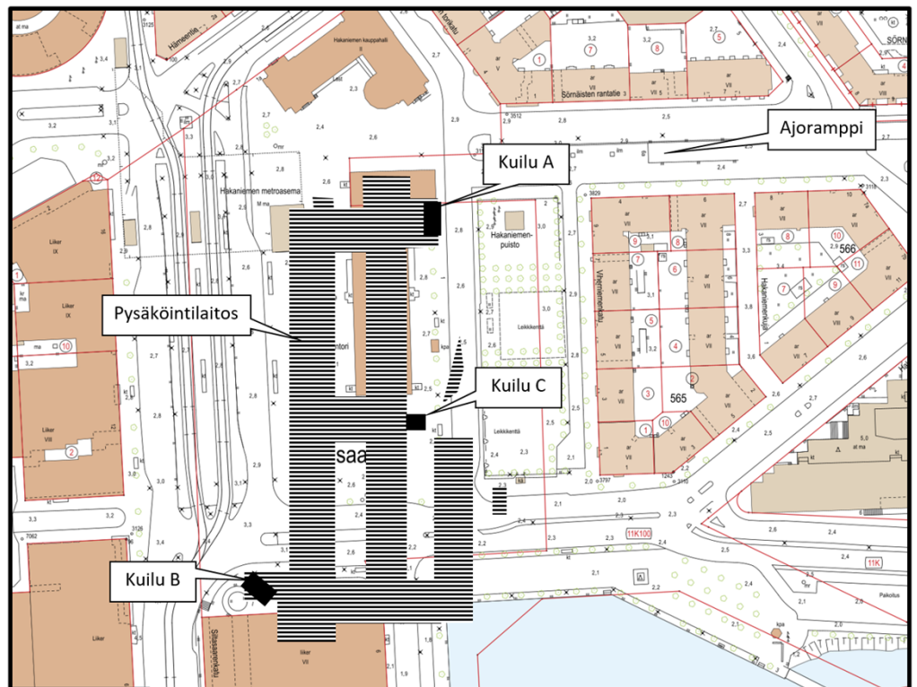
Kuva 1. Louhittavien pysäköintilaitoksen ja kuilujen sekä olemassa olevan ajorampin sijainnit.
