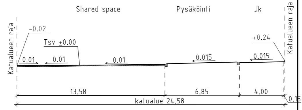
POIKKILEIKKAUS B-B 1:200
