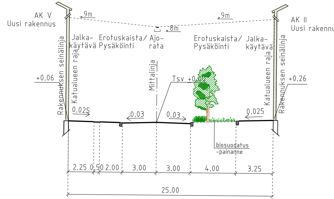
POIKKILEIKKAUS C-C
