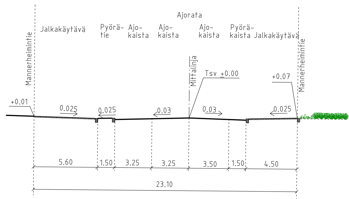
POIKKILEIKKAUS A-A
