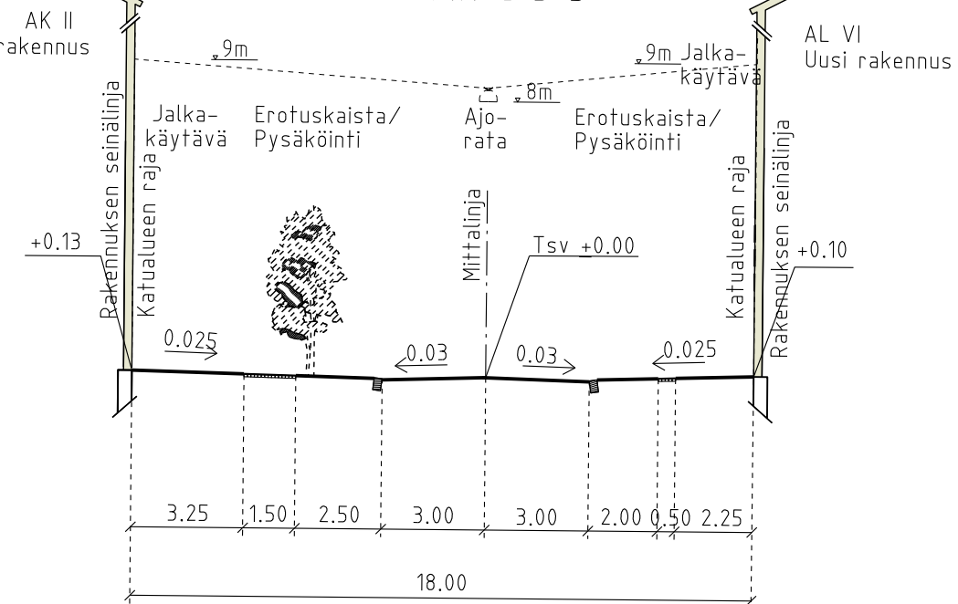
POIKKILEIKKAUS B-B
