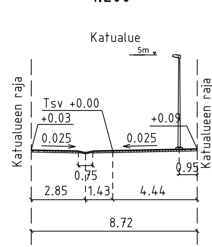
POIKKILEIKKAUS B - B 1:200
