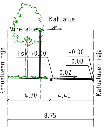
POIKKILEIKKAUS A - A 1:200
