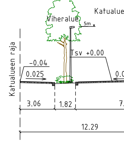
POIKKILEIKKAUS D - D 1:200
