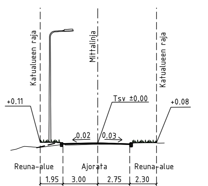
Leikkaus B-B 1:200
