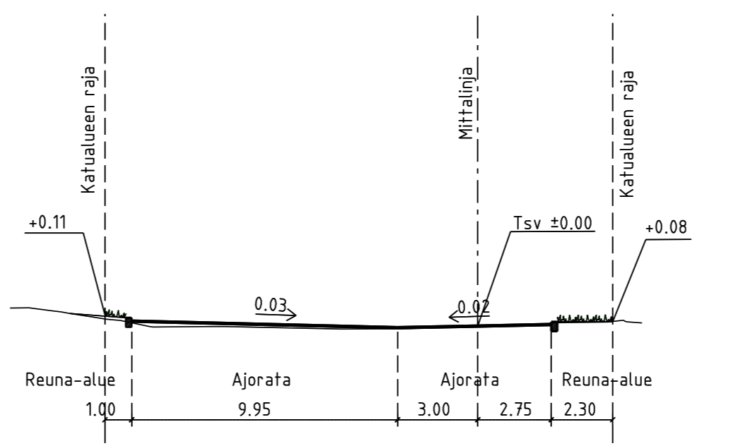
Leikkaus A-A 1:200
