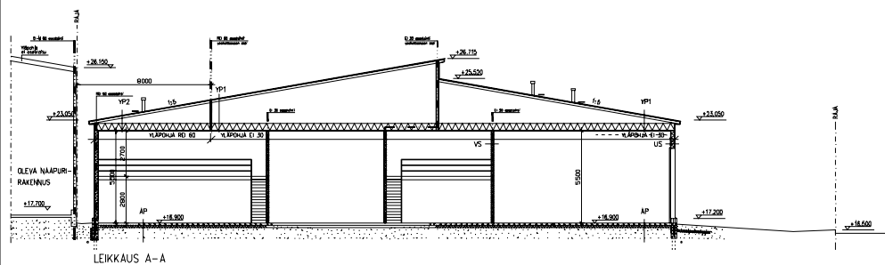
LEIKKAUS A-A
