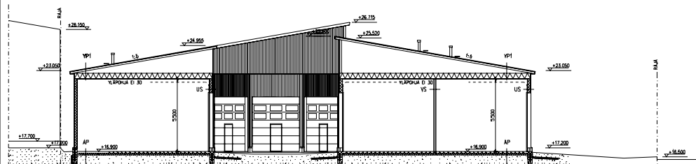
LEIKKAUS B-B
