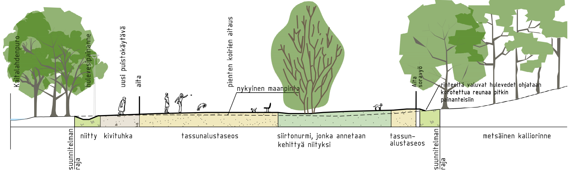
LEIKKAUS A-A' 1:200
