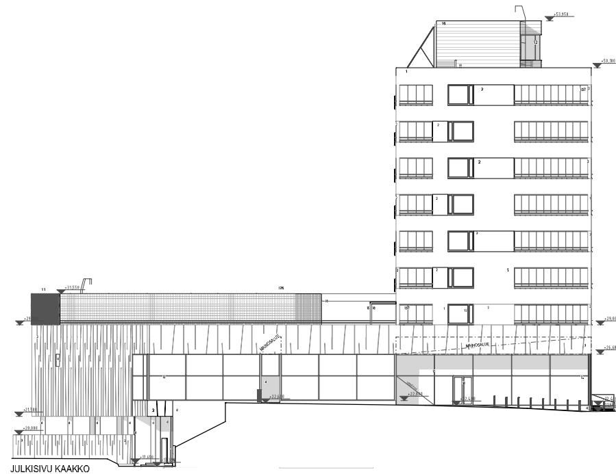
JULKISIVU KAAKKO
