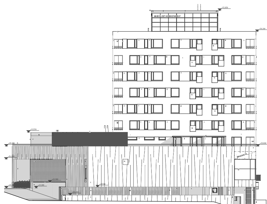
JULKISIVU LOUNAS
