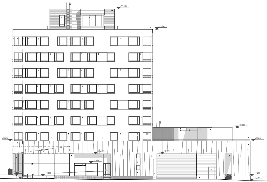
JULKISIVU KOILLINEN
