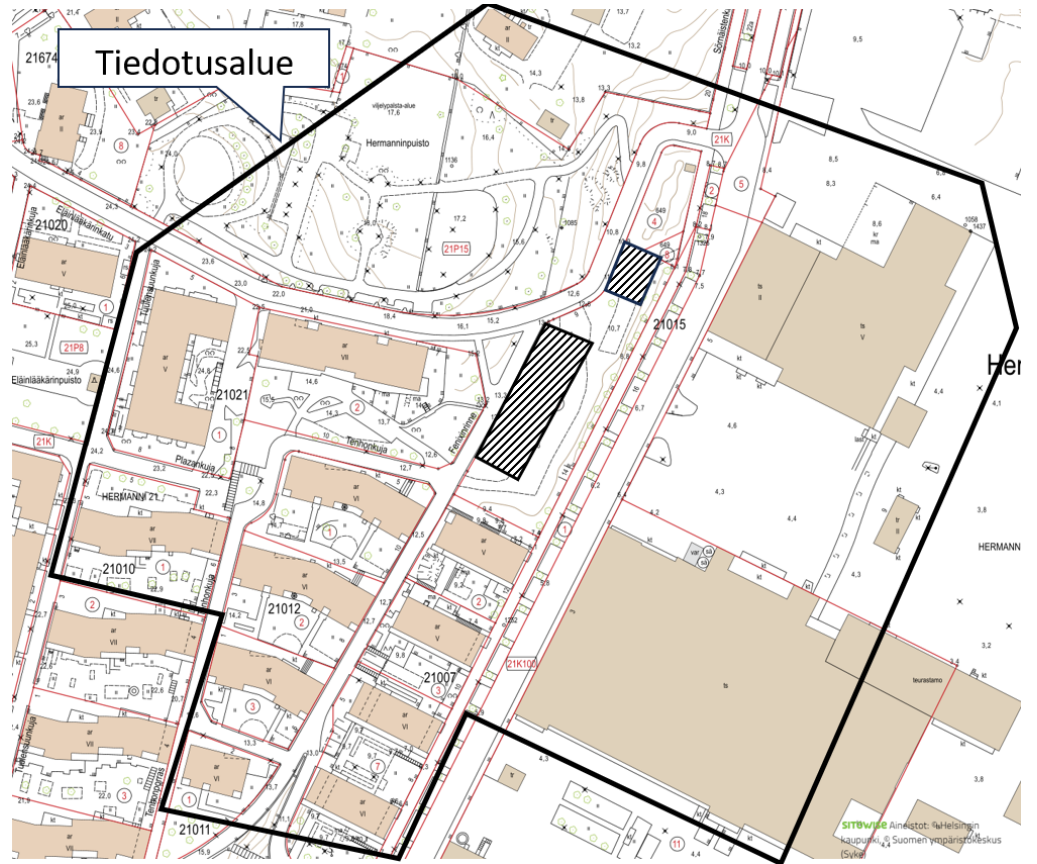
Kuva 1. Kartta tiedotusalueesta. Raudoitetuilla alueilla tehdään louhintaa, ponttausta ja paalutusta.
