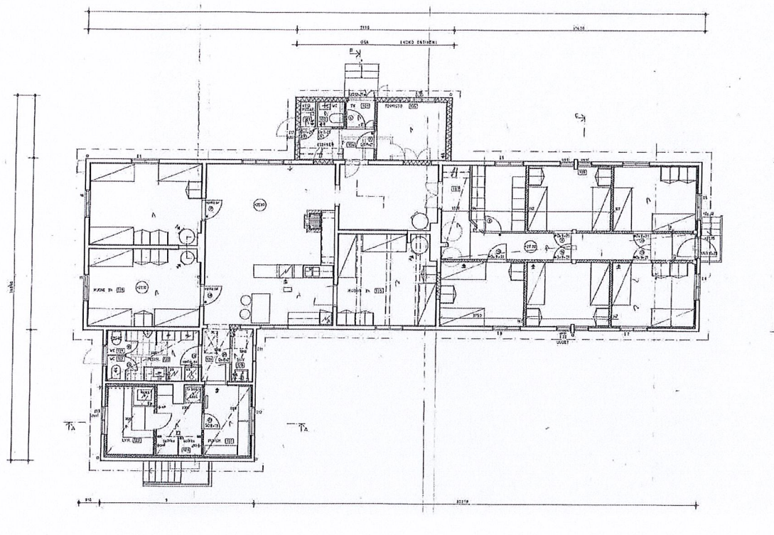
Kuva 5: Rakennus A, pohjapiirros lähtötilanteesta
