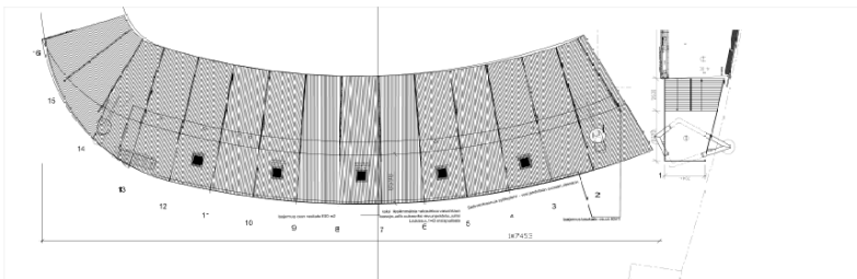
JULKISIVU PÖHJOISEN-TULEVA TILANNE MK 1/200
