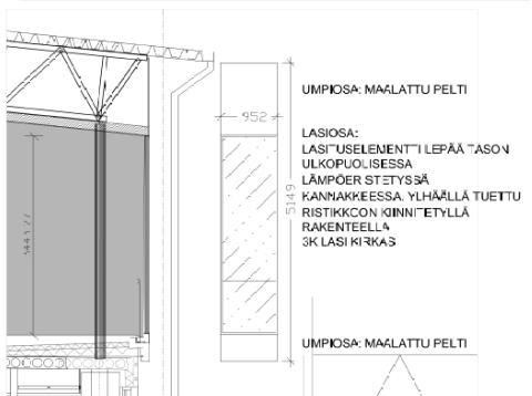
POIKILEIKKAUS MK 1/20
