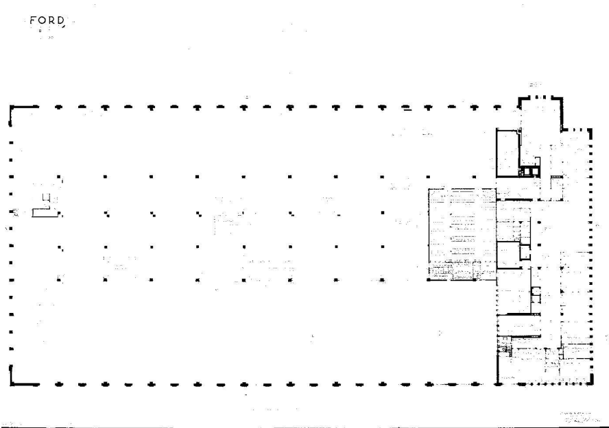
Kuva 4.11 Kokoonpanotehtaan 1. kerros, pääpiirustussarjan muutospiirustukset vuodelta 1945. Koy FORD
