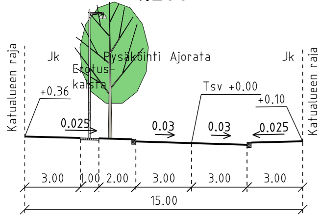
POIKKILEIKKAUS L-L 1:200
