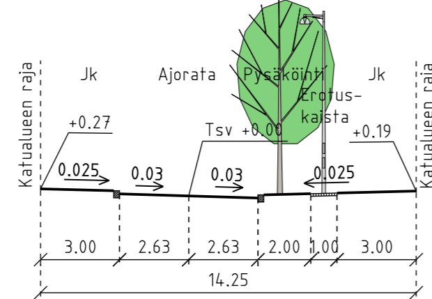
POIKKILEIKKAUS M-M 1:200
