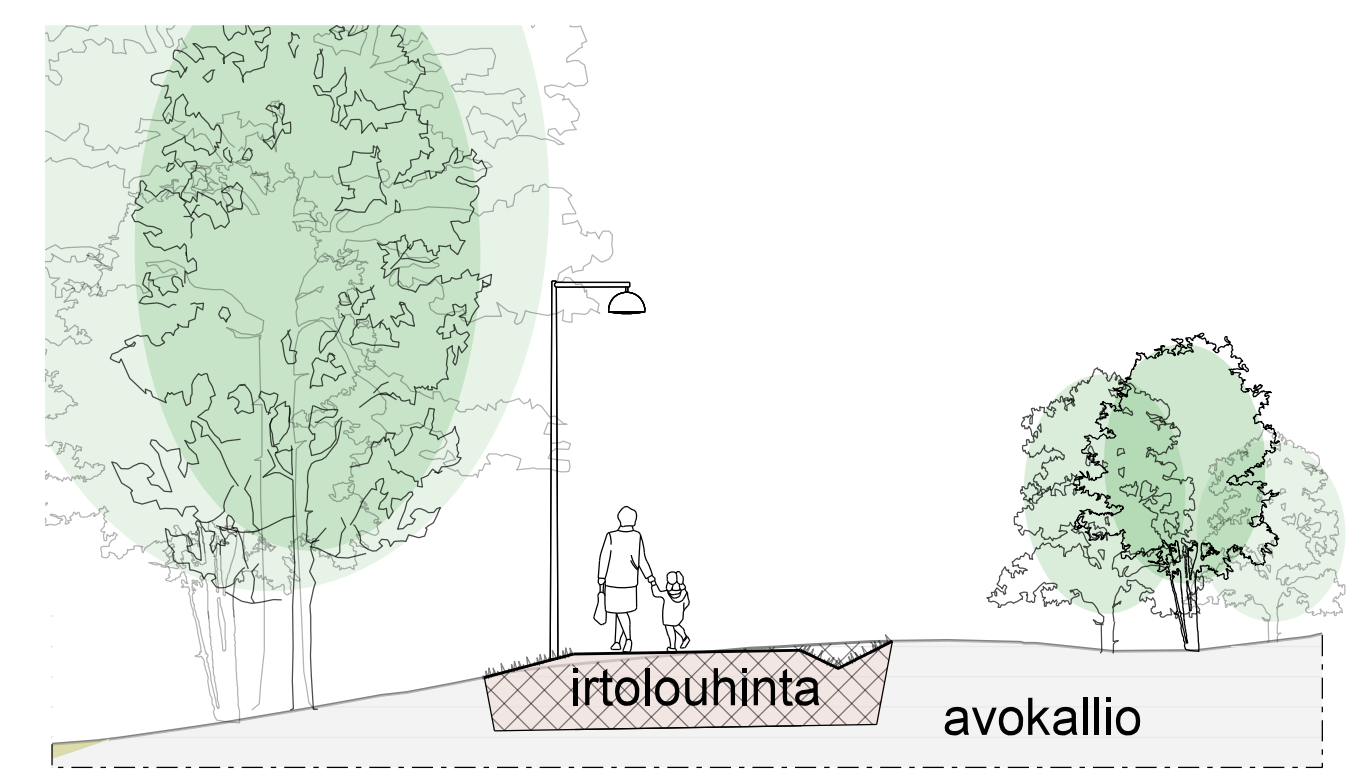
LEIKKAUS, 1:100 PAALU 40
