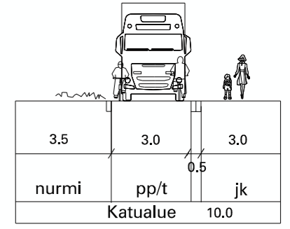
POIKKILEIKKAUS A - A
