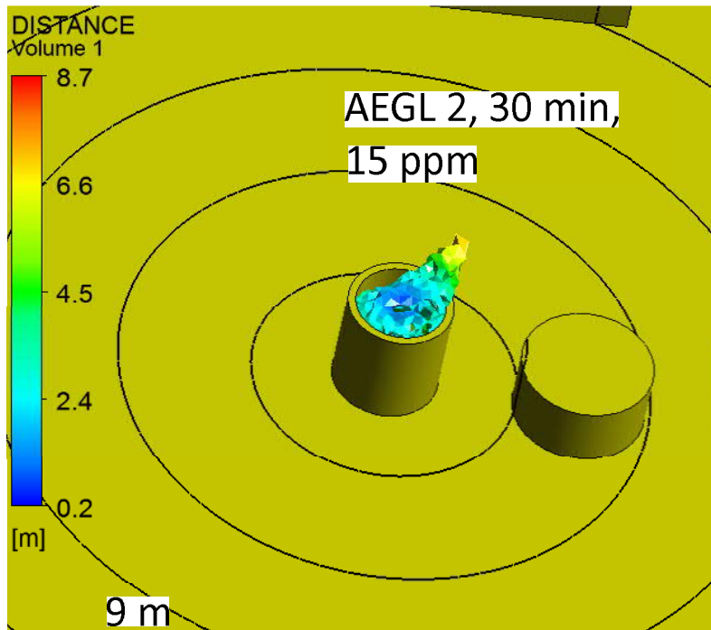
Kuva 16. Typpidioksidin leviämisalueet POK-säiliön palossa tuulen nopeudella 10 m/s, jolla AEGL-2 (30 min) pitoisuudet ylittyvät. AEGL-2 (10 min) ja AEGL-3 -rajat eivät ylitä.
