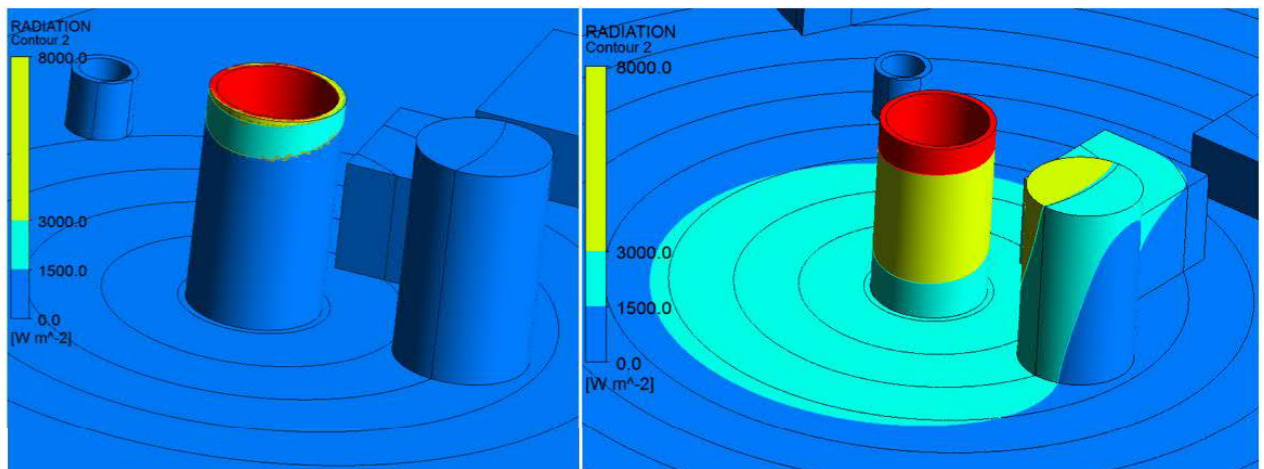
Kuva 12. Vertailu hakepalon lämpösäteilystä tuulen nopeudella 10 m/s, hakkeen kosteus 50 % ja 0 %.
