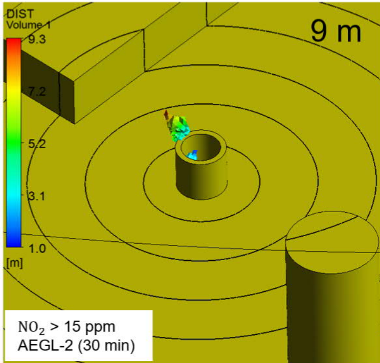
Kuva 19. Typpidioksidin leviämisalueet POK-säiliön palossa tuulen nopeudella 5 m/s, jolla AEGL-2 (30 min) pitoisuudet ylittyvät. AEGL-2 (10 min) ja AEGL-3 -rajat eivät ylity.
