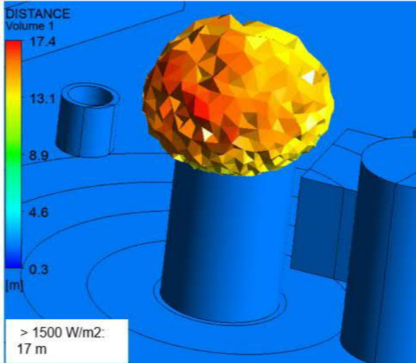
Kuva 13. Vertailu hakepalon lämpösäteilystä tuulen nopeudella 10 m/s, hakkeen kosteus 50 % ja 0 %.
