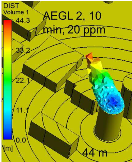
Kuva 26. Typpidioksidin leviämialueet hakepalossa tuulen nopeudella 10 m/s, joilla AEGL-2 ja AEGL-3 (10 min) pitoisuudet ylittyvät.
