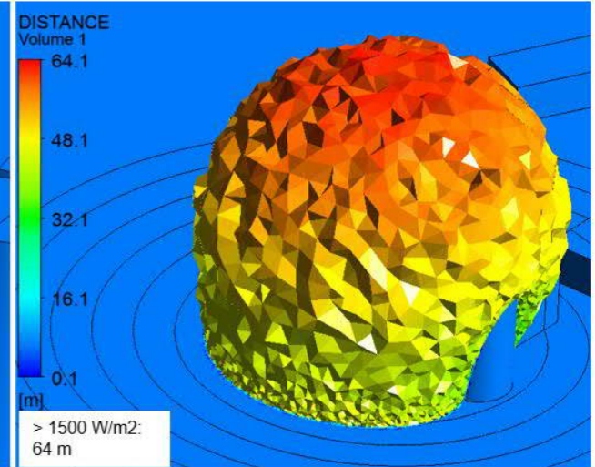
Kuva 13. Vertailu hakepalon lämpösäteilystä tuulen nopeudella 10 m/s, hakkeen kosteus 50 % ja 0 %.
