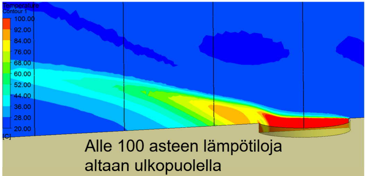
Kuva 41. Ammoniakkiliuossäiliön palon lämpötilat.
