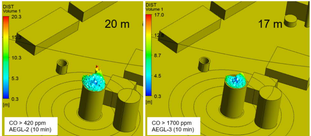
Kuva 28. Hiilimonoksidin leviämisalueet hakepalossa tuulen nopeudella 10 m/s, jolla AEGL-2 ja AEGL-3 (10 min) pitoisuudet ylittyvät.
