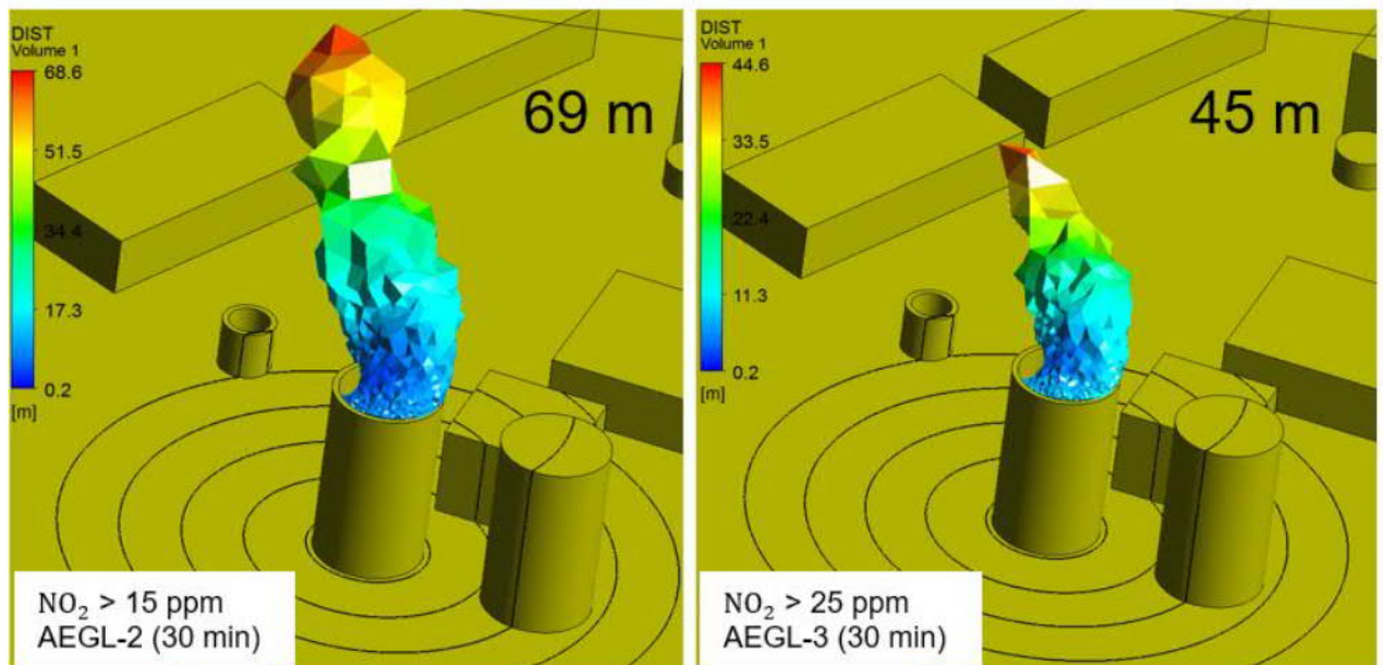
Kuva 29. Typpidioksidin leviämisalueet hakepalossa tuulen nopeudella 5 m/s, joilla AEGL-2 ja AEGL-3 (30 min) pitoisuudet ylittyvät.
