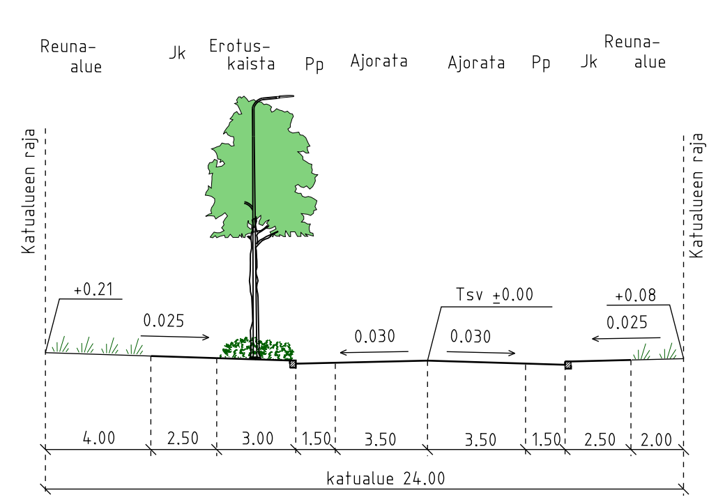
POIKKILEIKKAUS A - A 1:200
