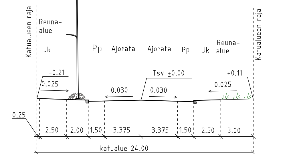
POIKKILEIKKAUS B - B 1:200
